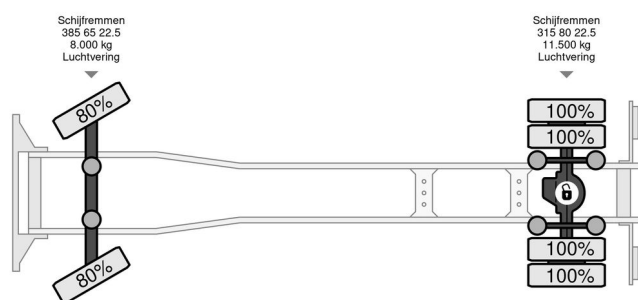
Scania G450 Scania G450 met Cuppers bak
