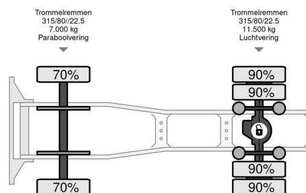
Scania R 143 MA 4x2 143 M
