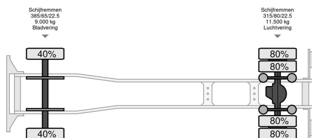
Scania P114-380 114G
