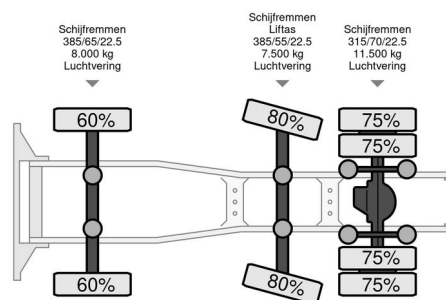
Scania R520 R520 6x2
