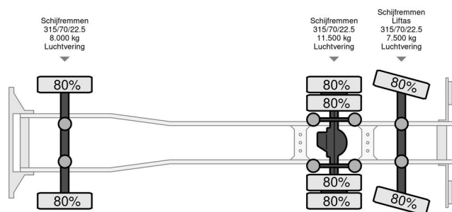
Volvo FH 460 FH 460
