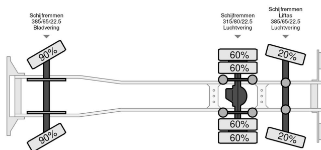
Volvo FH12 6X2R FAL8.0 RADT-A8 HIGH
