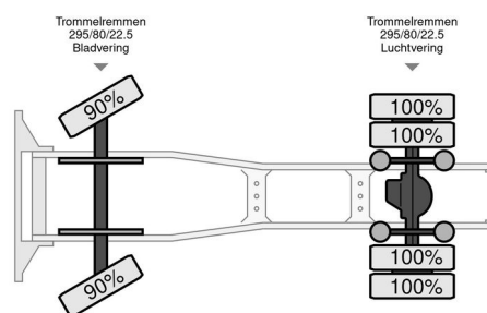
Mercedes-Benz Atego 1828 Atego 1828 LS - 1999
