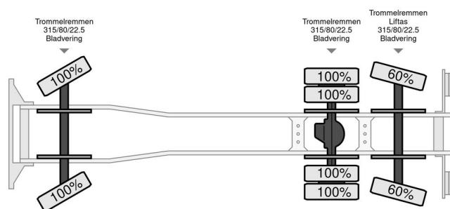
Volvo F 12 F12-20 6x2
