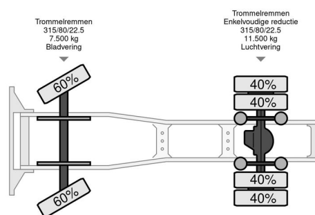
Scania R144-460 V8 144L - 460
