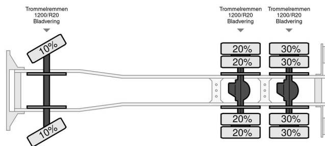
Mercedes-Benz SK 2632
