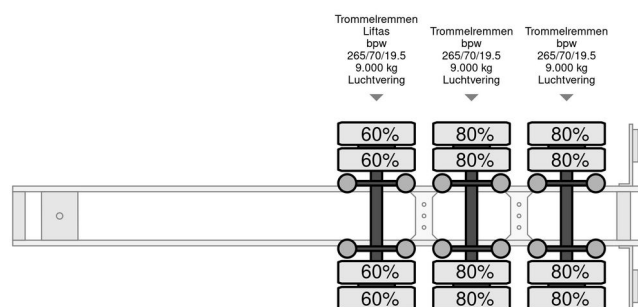
Pezzaioli SBA32
