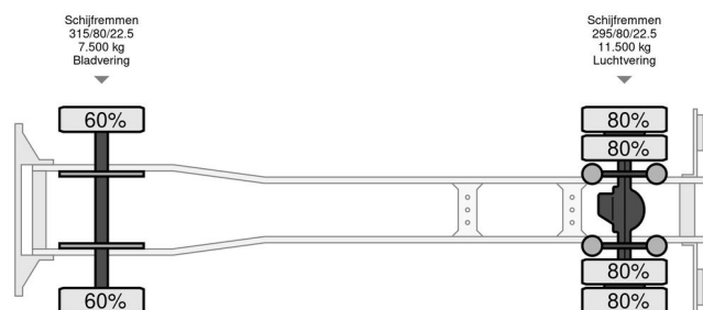
Scania P114-340 P114
