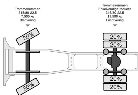
Scania R143-500 V8 met nieuwe APK - with new MOT - Mit neuem TuV 4x2 Referentienummer: 79BVD4
