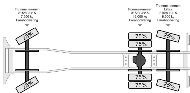
Volvo F 12 F12 6x2
