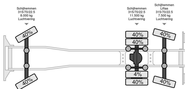
Volvo FH 460 FH 460
