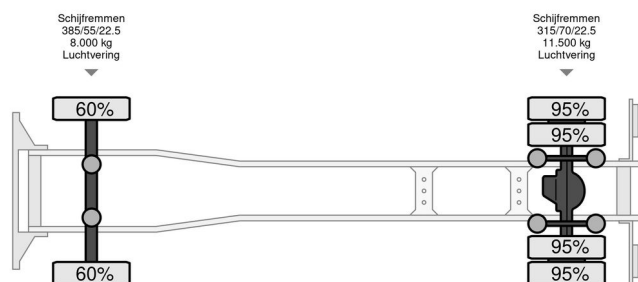
Scania G450 G450 - Topline
