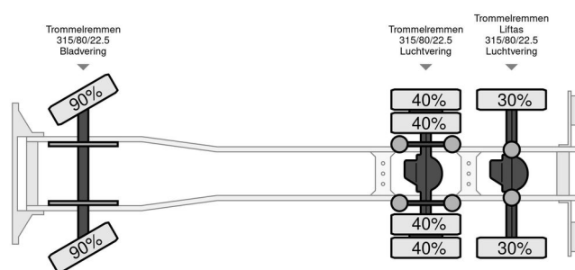
Scania R143-450 V8 143-450
