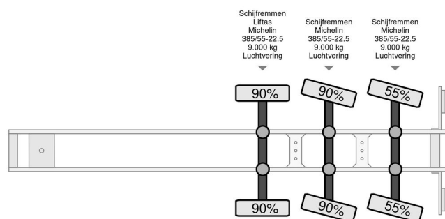
Van Hool Bekkers Type 1 92.10 m2
